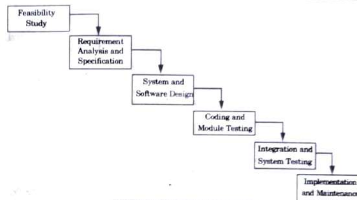
Fig. 1.12.1. Waterfall model.
