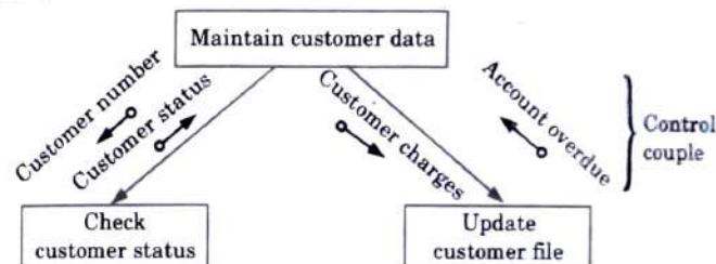
Fig. 3.7.1. Structure chart.
